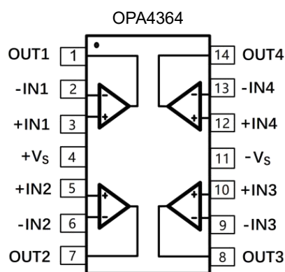
SOP-14/TSSOP-14
