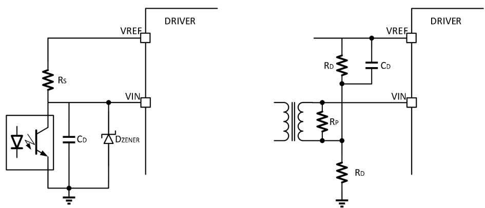
图 9-9 输入端光电耦合器或脉冲变压器
