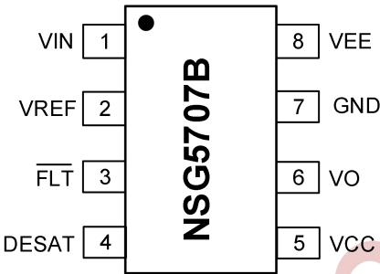
图 6-1 8-脚 SOP8 顶视图
