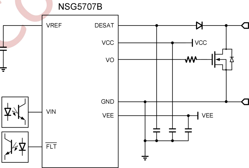
图 9-2 NSG5707B 典型应用电路图
