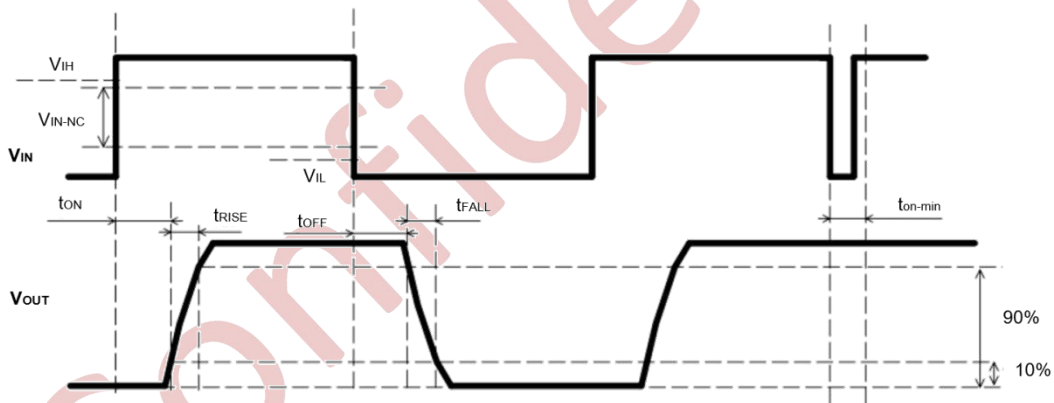
图 9-11 光电耦合器输入和输出信号参数
