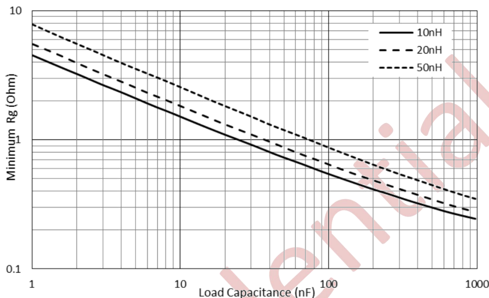
图 9-4 随 IGBT/MOSFET 栅极电容变化的推荐最小栅极电阻
