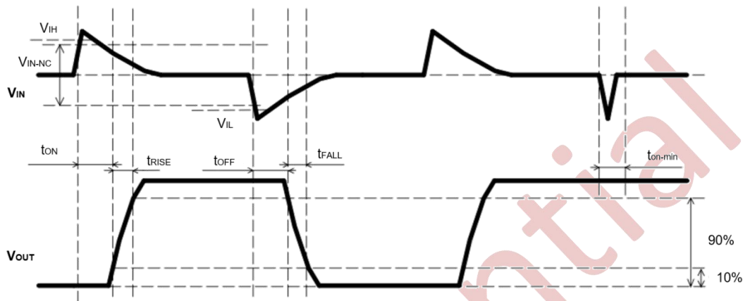
图 9-10 脉冲变压器输入和输出信号参数
