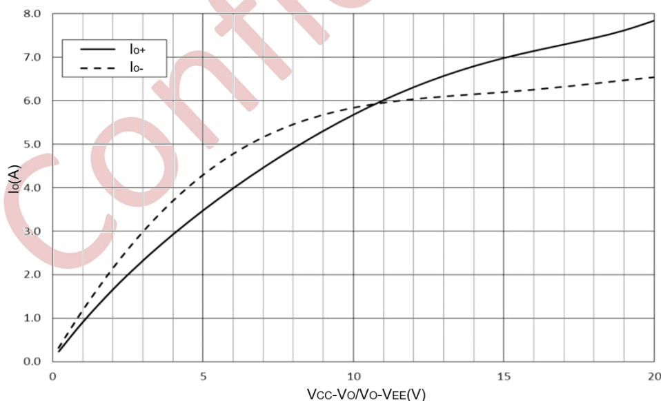
图 9-3 输出电流与输出电压降的关系
