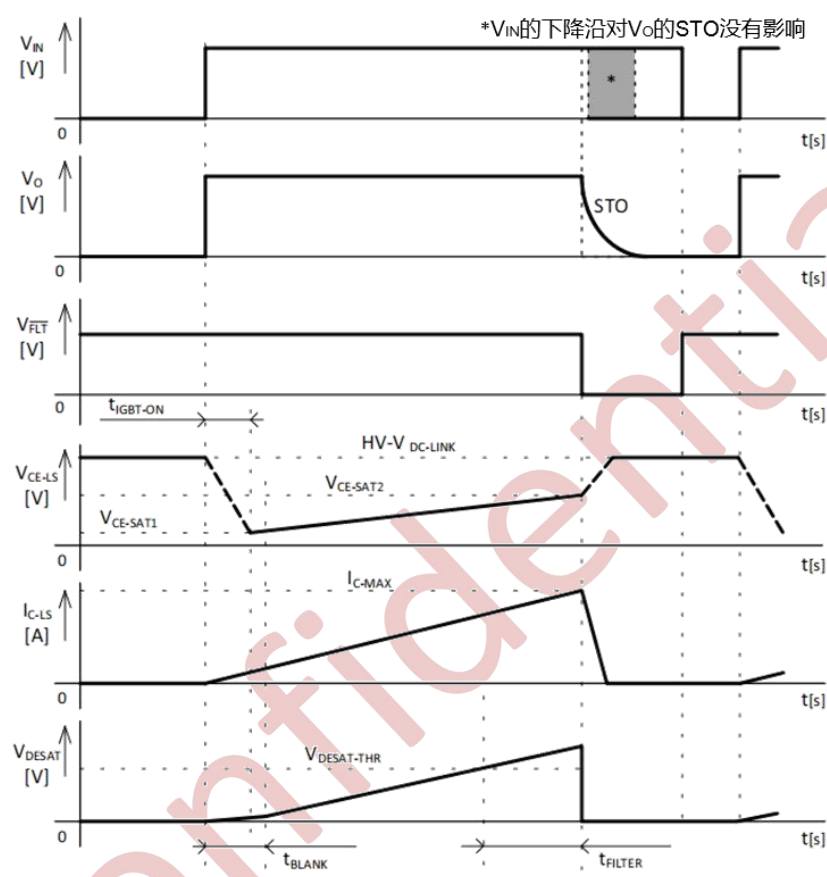
图 9-8 DESAT 保护波形
