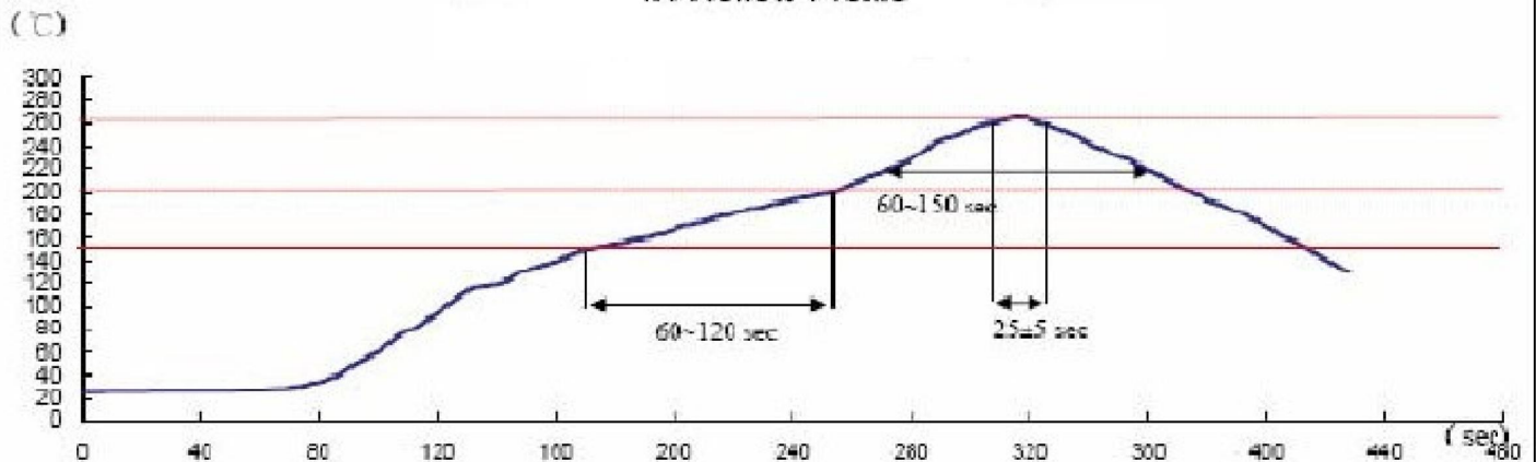
IR-Reflow Profile
