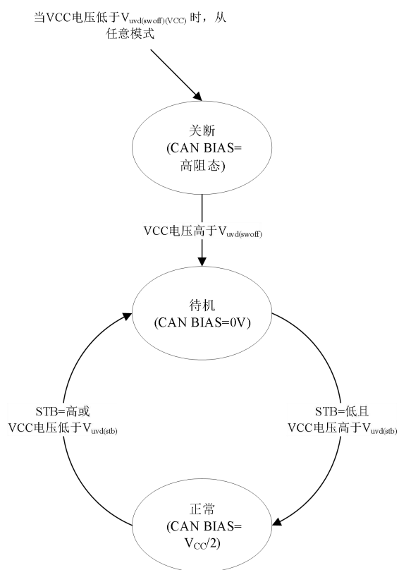
图 8 SIT1044GQ 状态图
