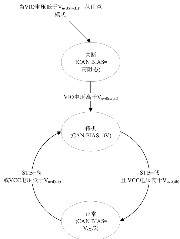
图 7 SIT1044GQ/3 状态图
