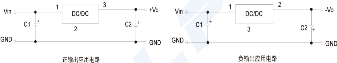
图 2 典型应用电路
