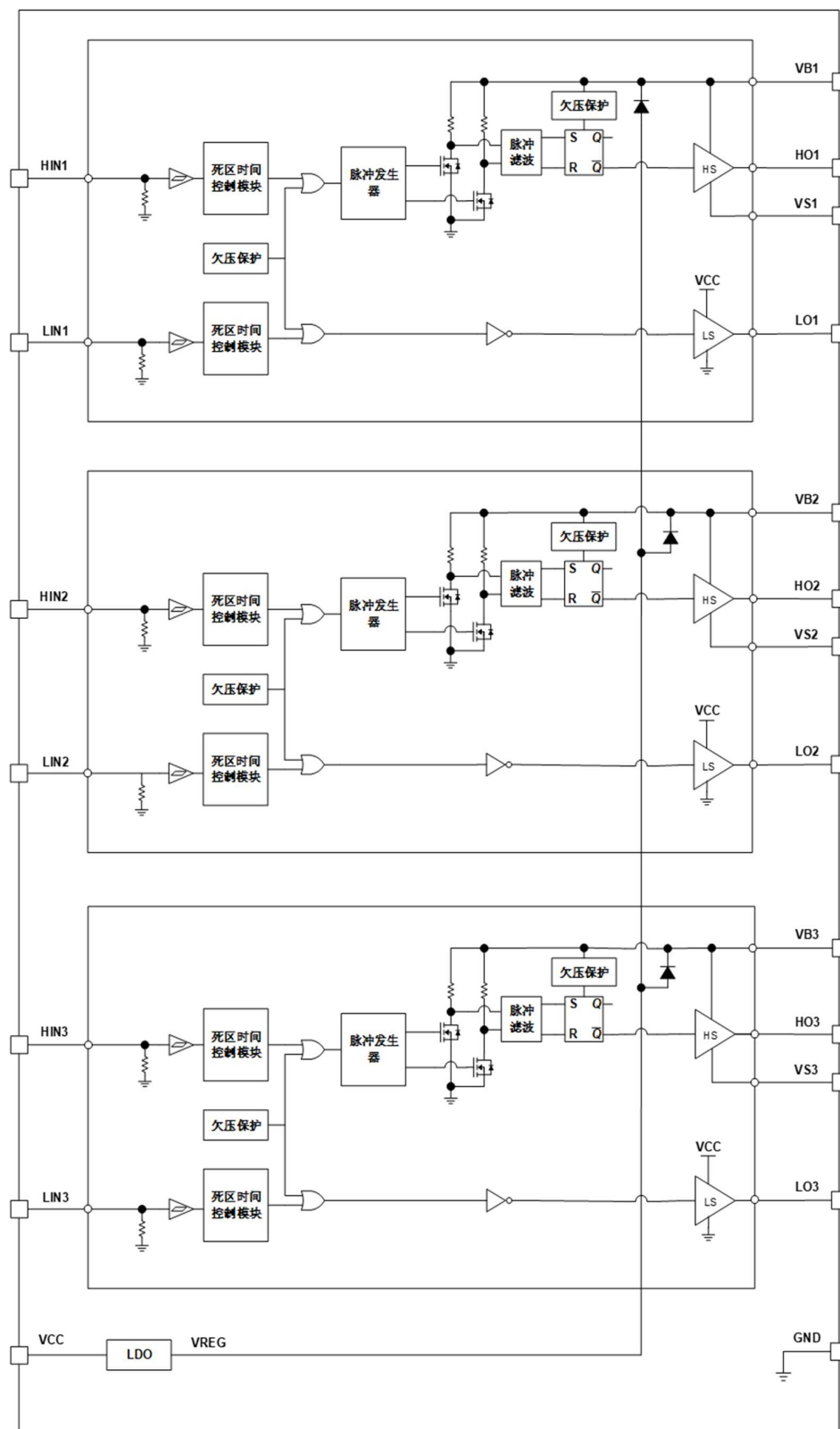
图 1. HT6288A 功能框图
