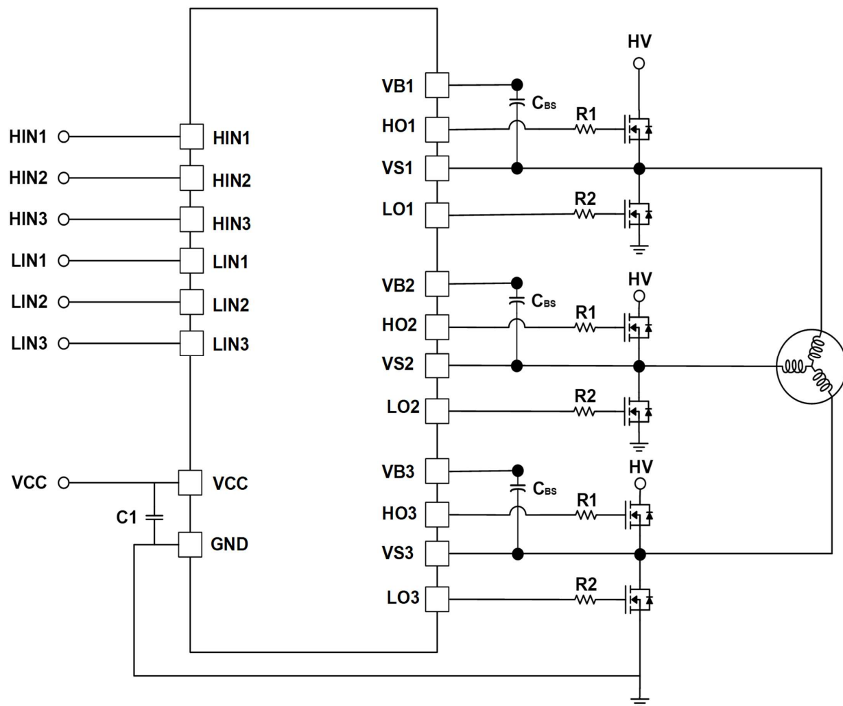
图 2. 无刷电机驱动参考电路
