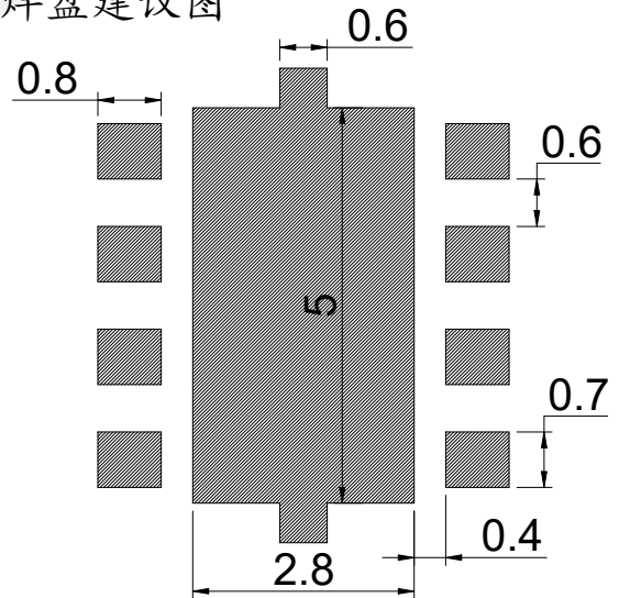
焊盘建议图
