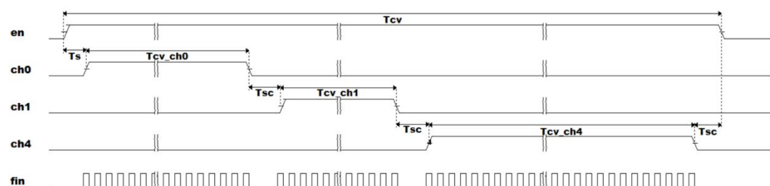
图 8.4-1 测量工作流程
