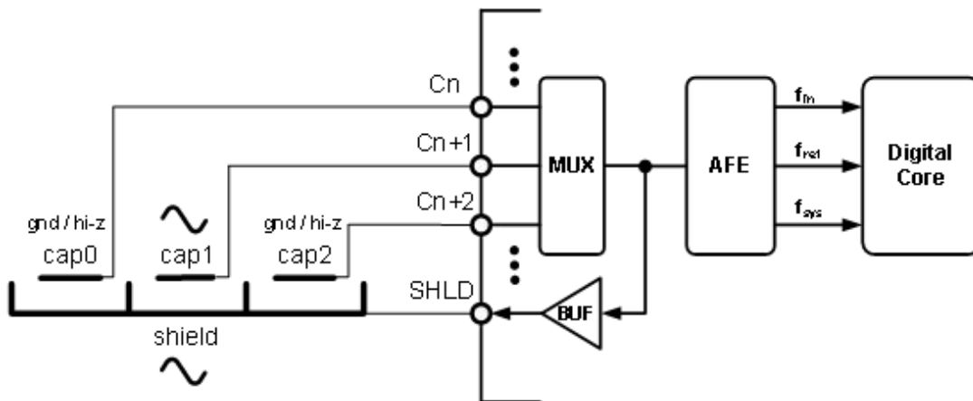
图 8.9-1 模式 1-单路有源屏蔽
