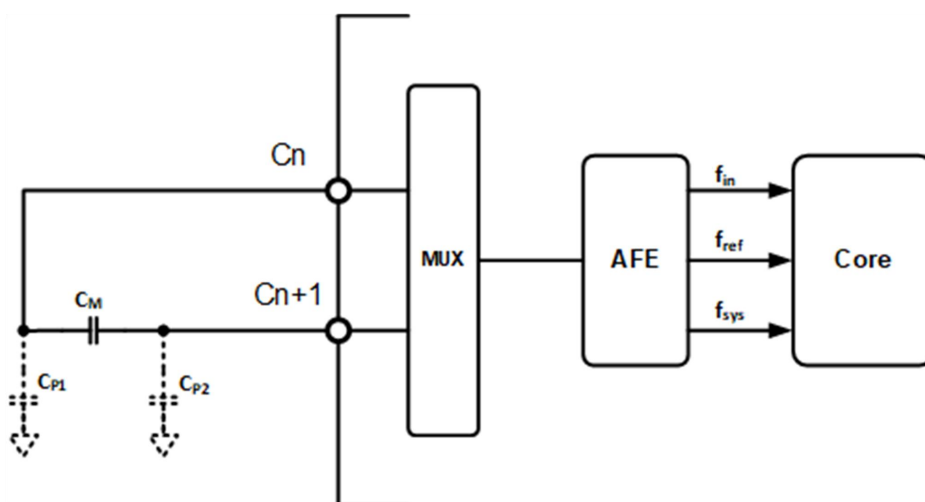
图 8.3.3-1 测量互电容
