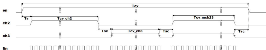
图 8.4-2 互电容测量工作流程
