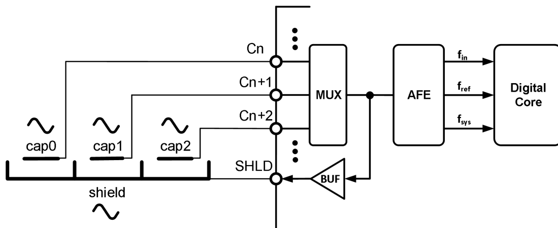
图 8.9-2 模式 2-多路有源屏蔽
