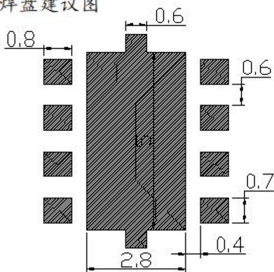
焊盘建议图
