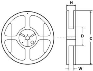
Reel Dimensions 卷盘规格
