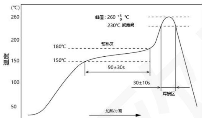
回流焊曲线图
