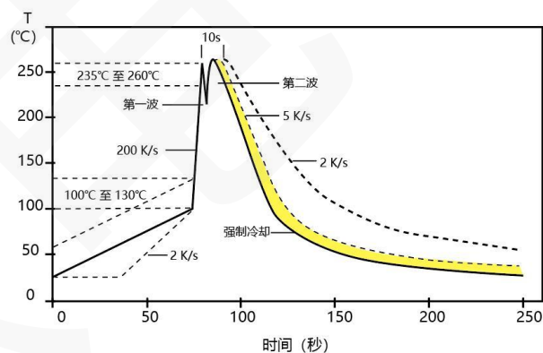
波峰焊曲线图
