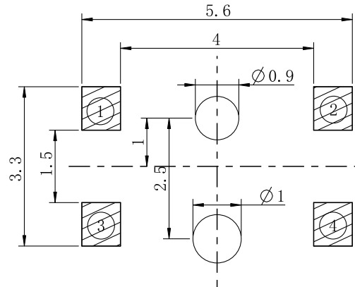
焊接图
