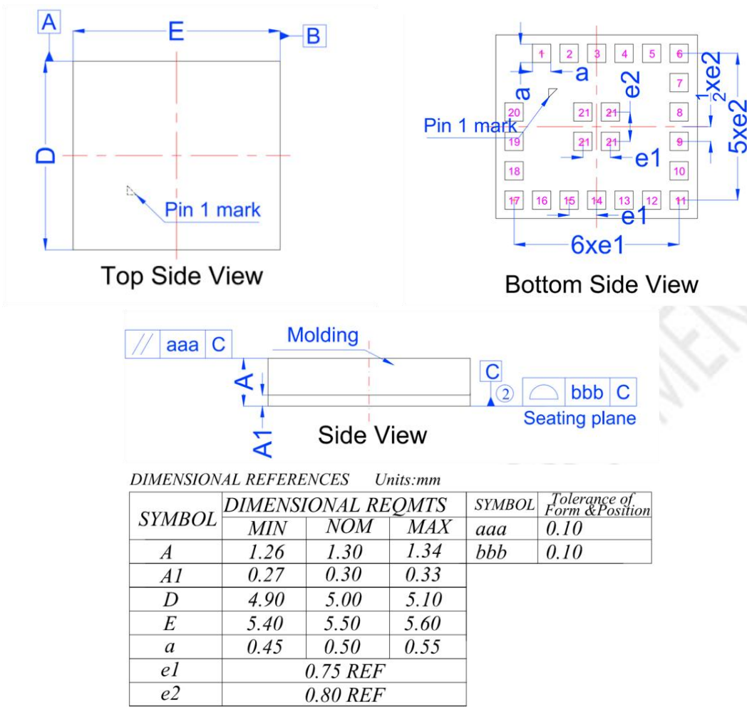
图 6. 1： HJ-180IMH-15 机械尺寸图
