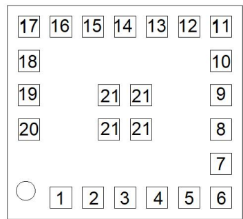
图 2.2：HJ-180IMH-15 引脚分布图（正面图）
