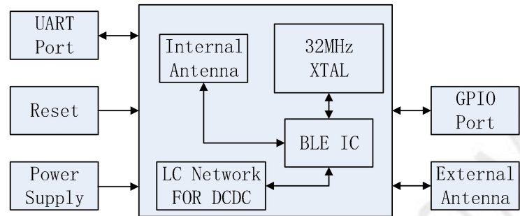
图 2.1：HJ-180IMH-15 功能框图
