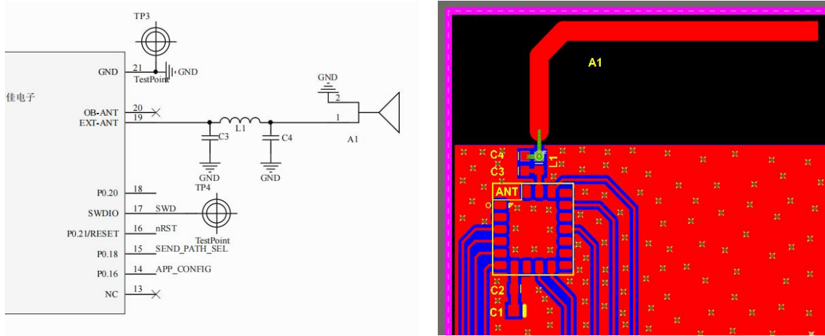
图 3.2：使用外接天线
