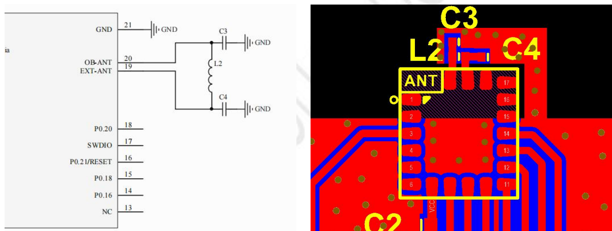
图 3.1：使用模组内置天线
