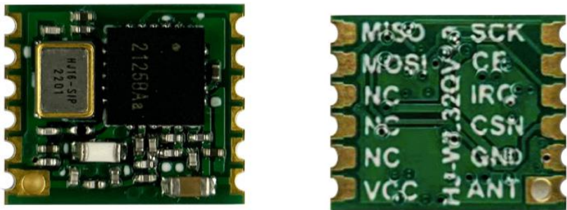
图 1.1：HJ-WL32Q 正面和底面图
