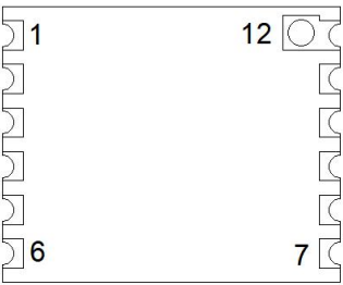
图 2.2：HJ-WL32Q 引脚分布图
