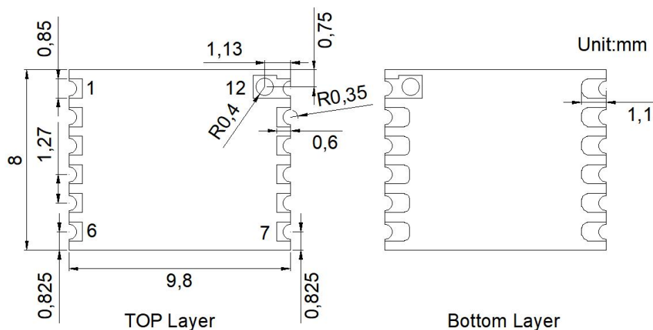
图 6.1: HJ-WL32Q 机械尺寸图
