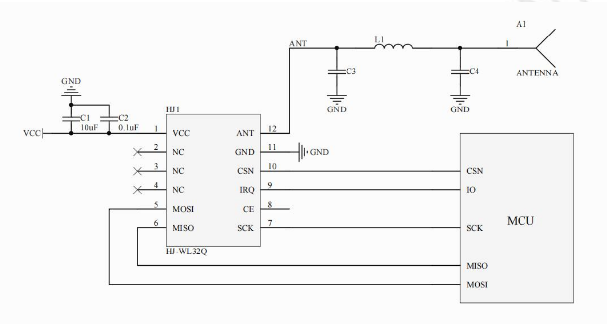
图 5.1：参考原理图
