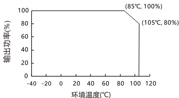
温度曲线图
