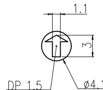
ACTUATOR
