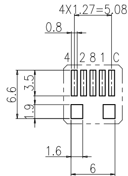
P.C.B DIMENSION
