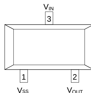
SOT23-3
