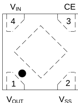
FBP4L(1.0*1.0*0.37-0.65) DFN4L(1.0*1.0*0.37-0.65)
