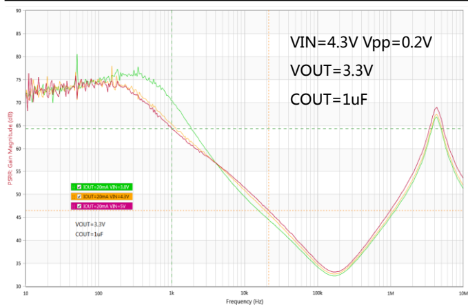
图 11. 纹波抑制比与频率
