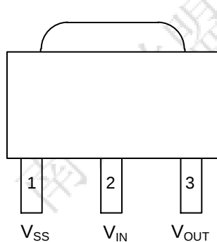
SOT89-3
