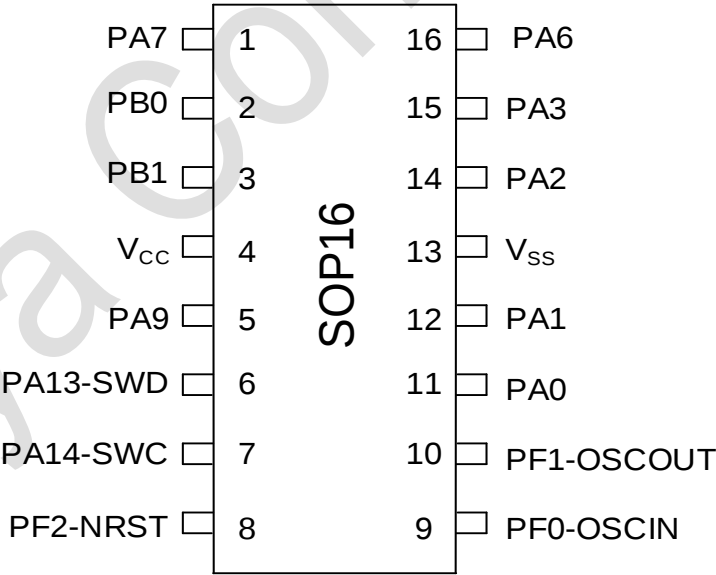
图 3-4 SOP16 Pinout1 PY32F002AW15Sx
