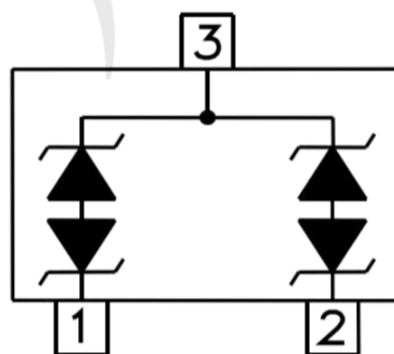
SOT-323
