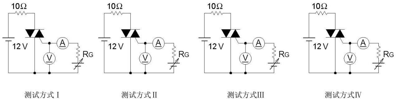
图九、门极触发特性测试电路
