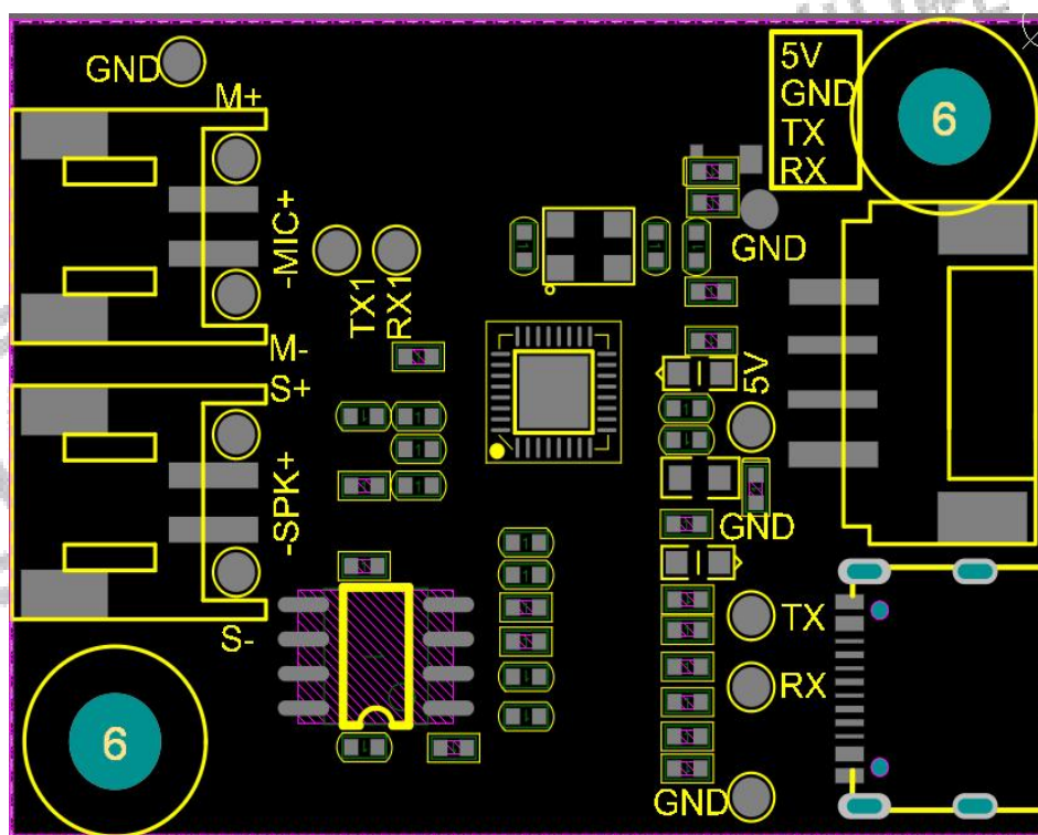
图表 10- WTK6900HC-32N M02 V3.02 模块封装管脚图
