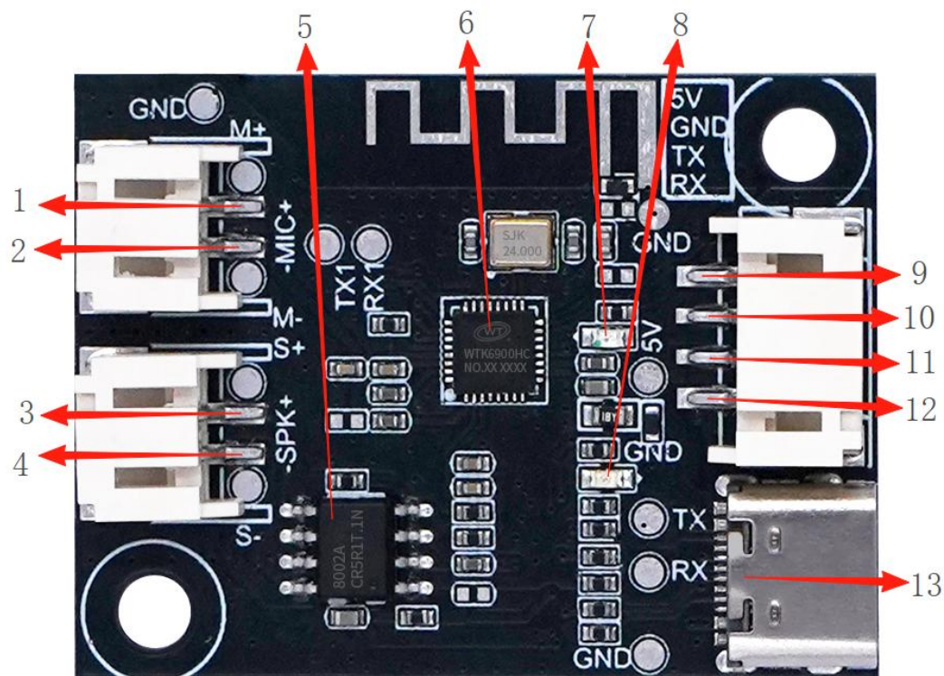
图表 8- WTK6900HC-32N M02 V2.02 模块实物图
