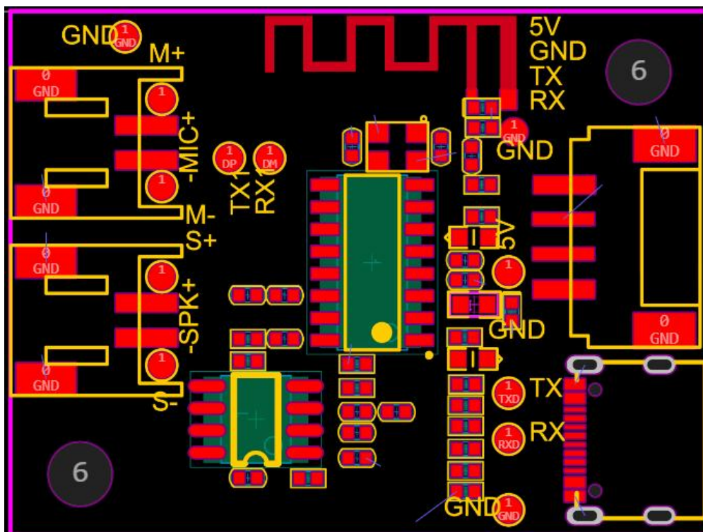
图表 4- WTK6900HC-16S M02 V2.02 模块管脚封装图
