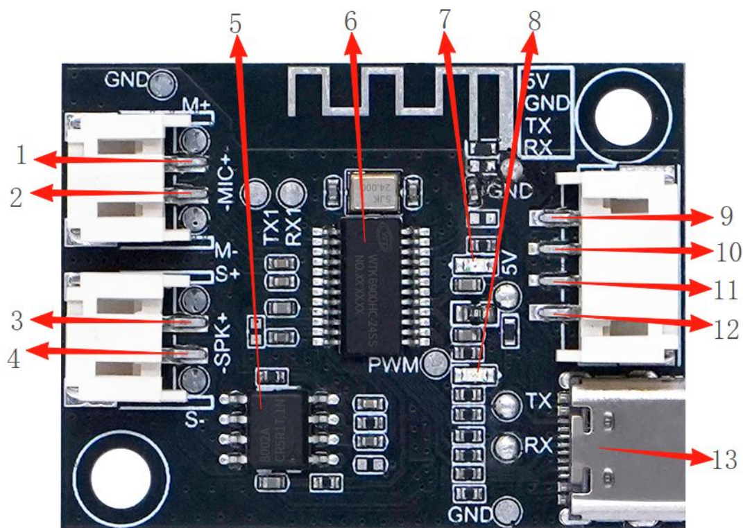
图 5- WTK6900HC-24SS M02 V2.02 模块实物图
