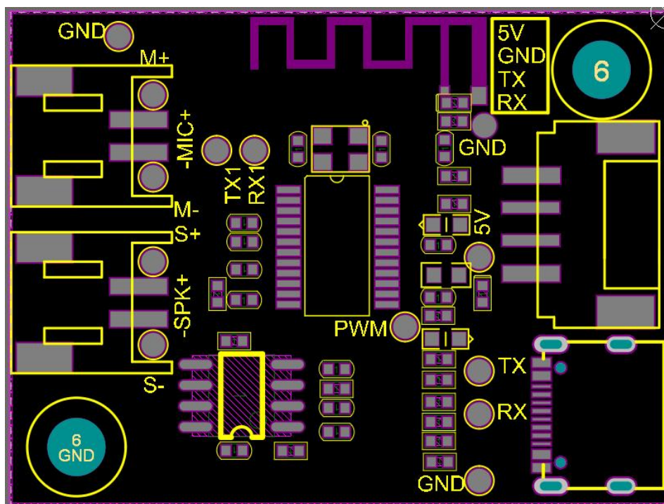
图表 7- WTK6900HC-24SS M02 V2.02 模块封装管脚图
