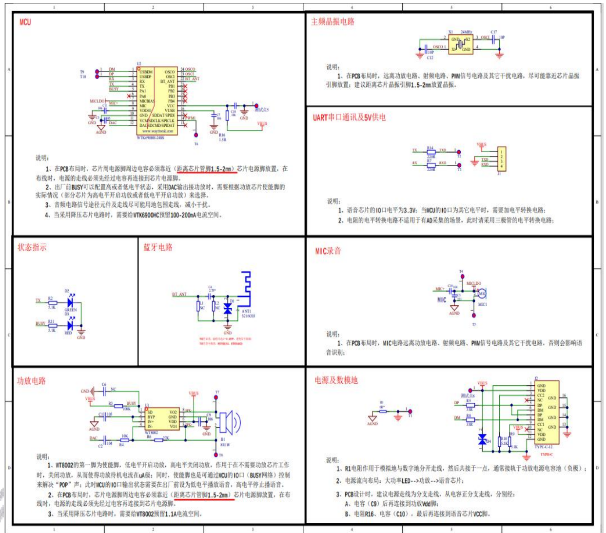
图表 13- WTK6900HC-24SS M02 V2.02 电路设计参考图
