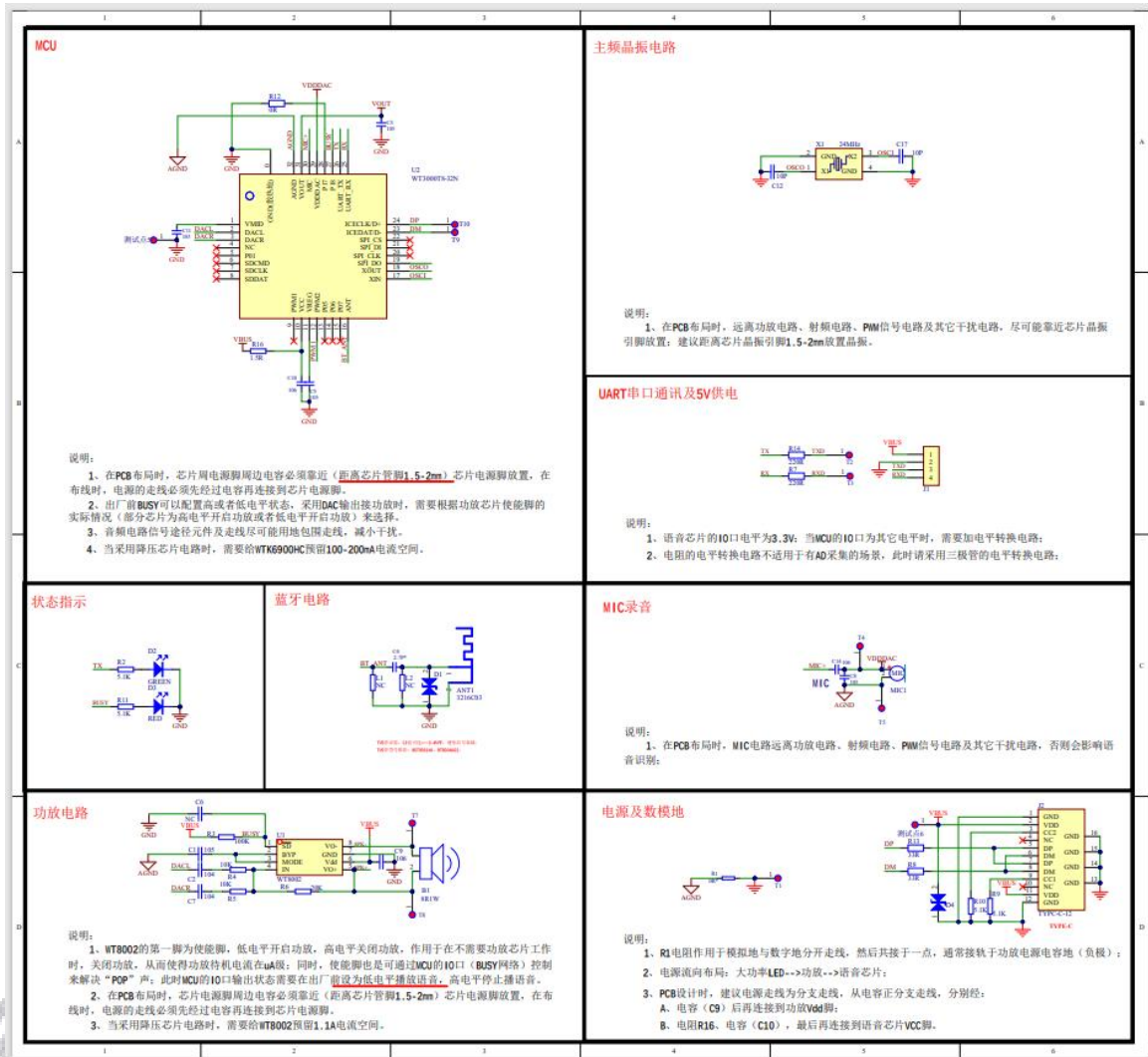
图表 14- WTK6900HC-32N M02 V3.02 电路设计参考图
