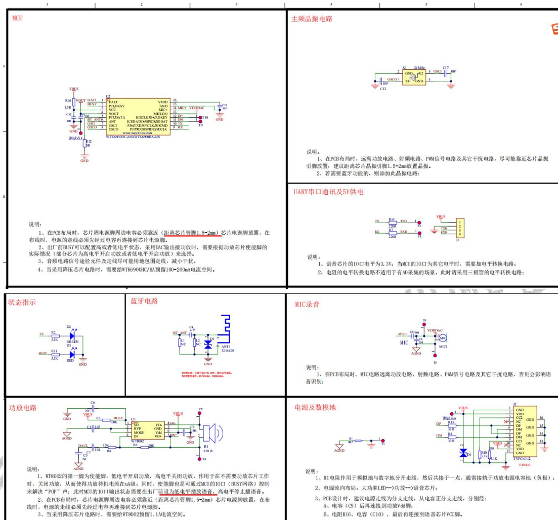
图表 12- WTK6900HC-16S M02 V1.03 电路设计参考图
