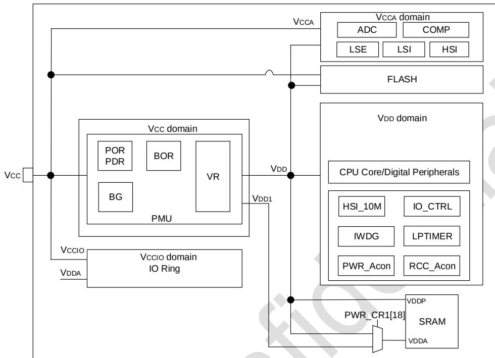
图 2-2 电源框图
