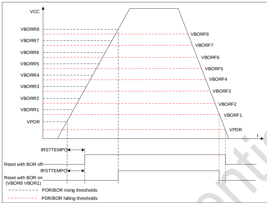
图 2-3 POR/PDR/BOR 阈值
