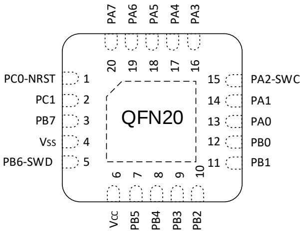
图 3-1 QFN20 Pinout1 PY32C642F15U6-C
