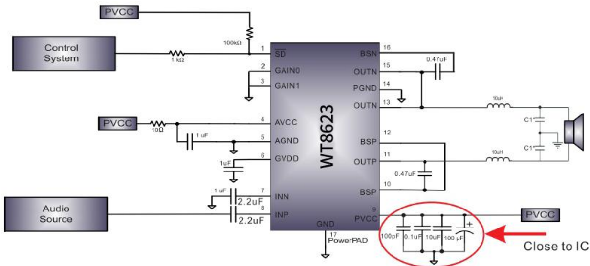
单端输入应用线路图
