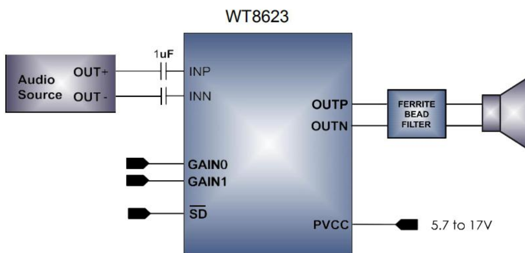
差分输入应用线路图
