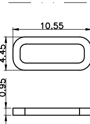
防水圈图示
