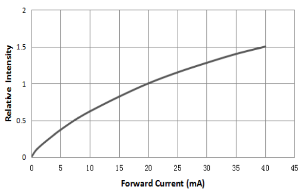
相对光强与电流特性曲线
