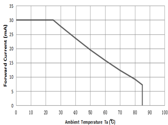
最大正向电流与环境温度特性曲线
