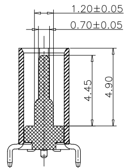
SECTION A-A SCALE 1:1
