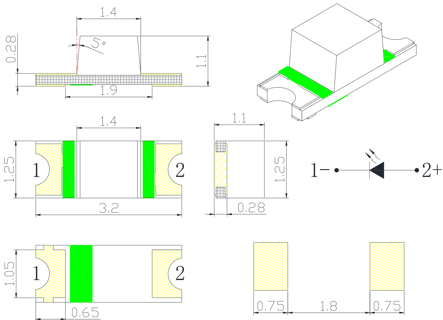
建议焊盘尺寸
