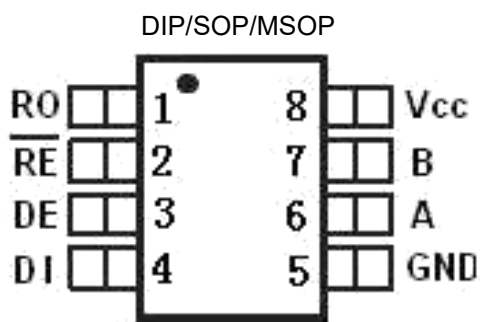
图 2: SNx5176 引脚图
