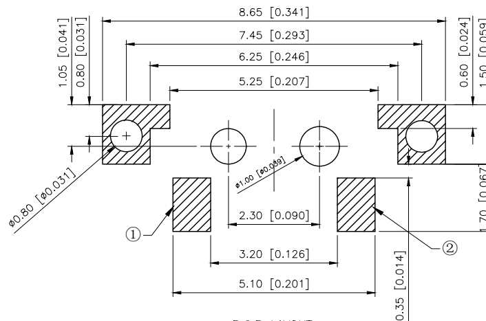
P.C.B LAYOUT
