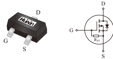
SOT-23
