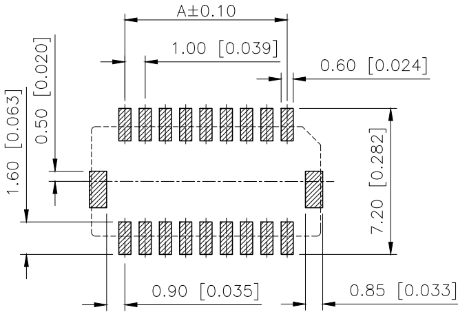
P.C.B Layout
