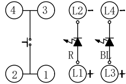
电原理图
