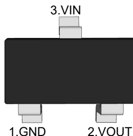
SOT-23-3
