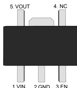
SOT-89-5
