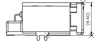
8~12 PIN
