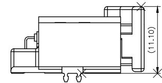
16~20 PIN
