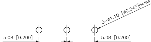
P.C.B LAYOUT
