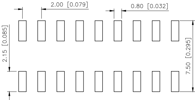
P.C.B LAYOUT
