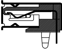
剖面 A-A 比例 1:1
