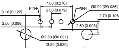
PCB 孔位图
