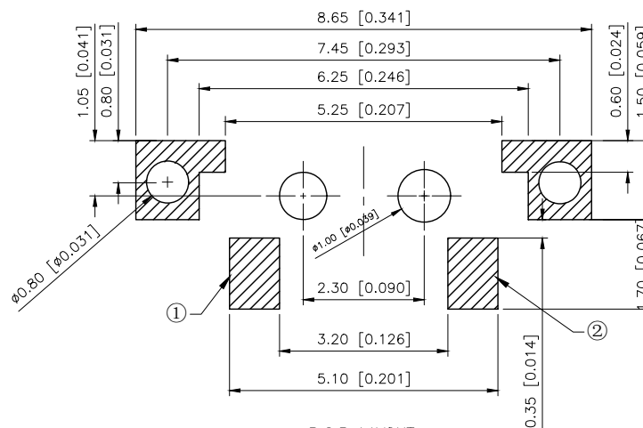
P.C.B LAYOUT
