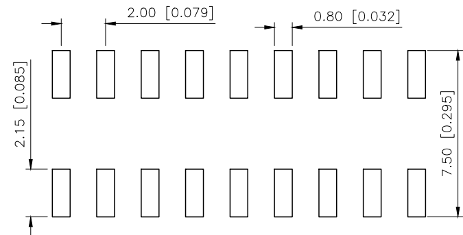
P.C.B LAYOUT
