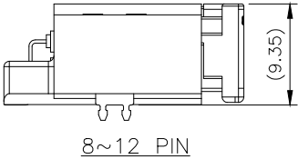
8~12 PIN
