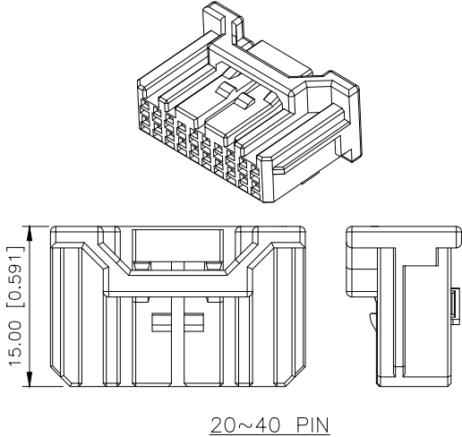
20~40 PIN
