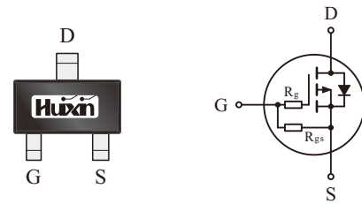
SOT-523
