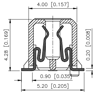
SECT:A-A 2:1
