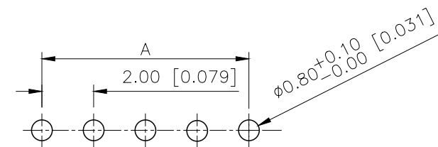
P.C.B LAYOUT
