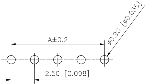
P.C.B LAYOUT
