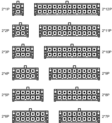
Scale 1:3
