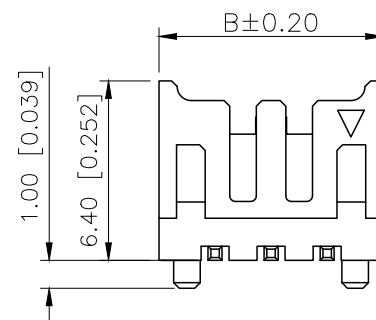
2P视图
