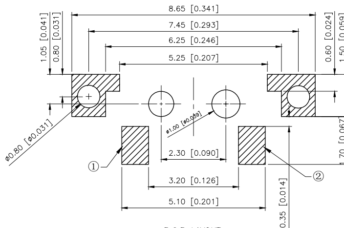
P.C.B LAYOUT
