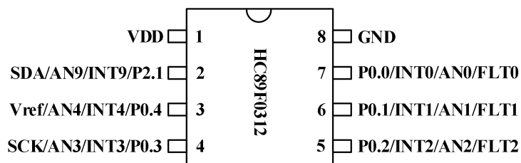
Figure 1-4 SOP8 引脚配置图
