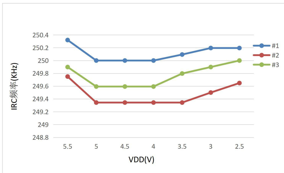
Figure 22-3 内部高频 RC32M/128-电压特性曲线图
