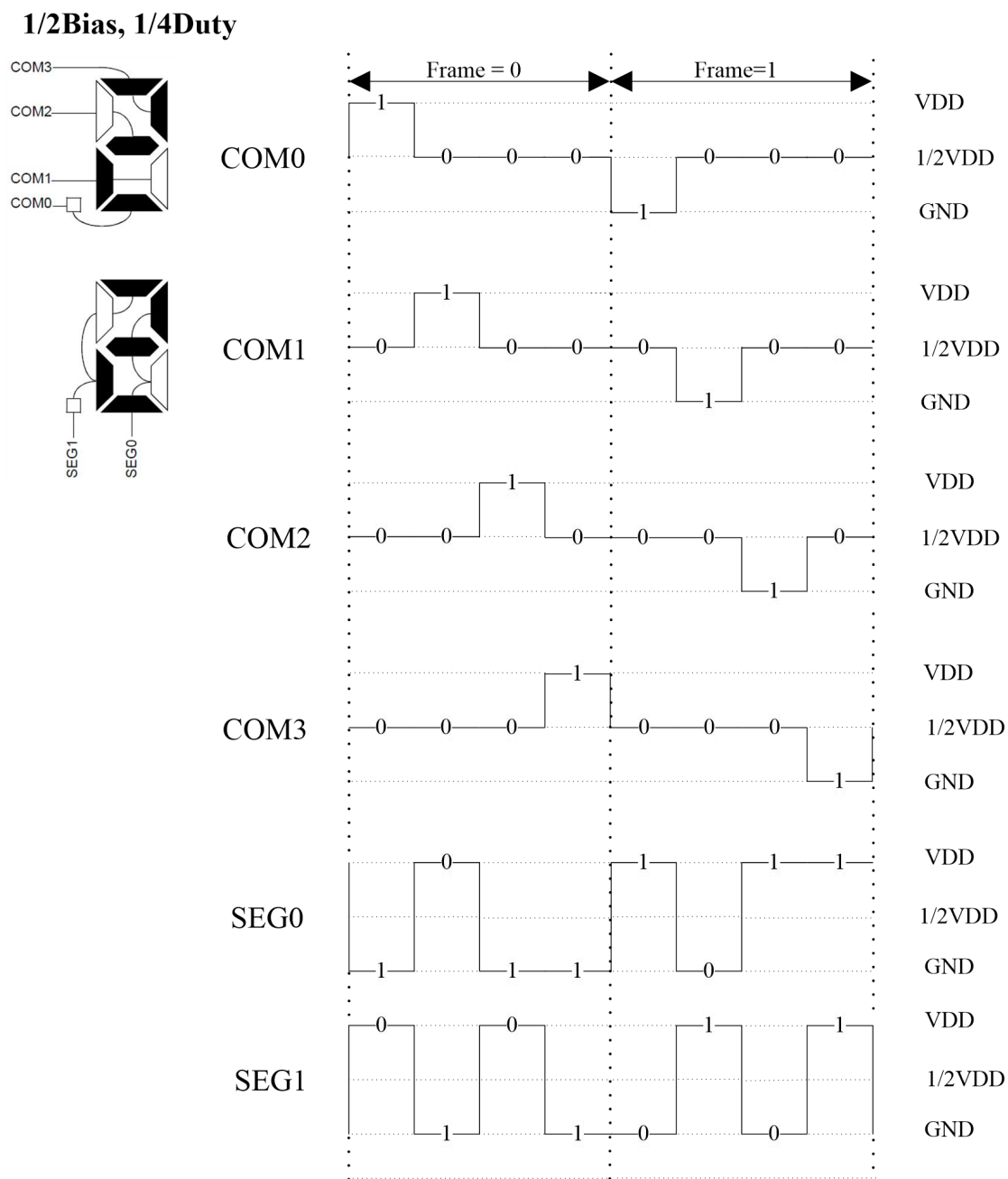
Figure 17-2 1/2bias LCD 波形图
