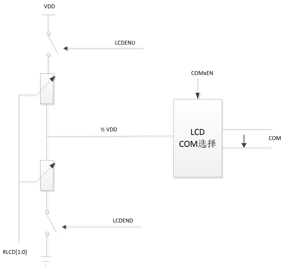
Figure 17-1 LCD 系统框图
