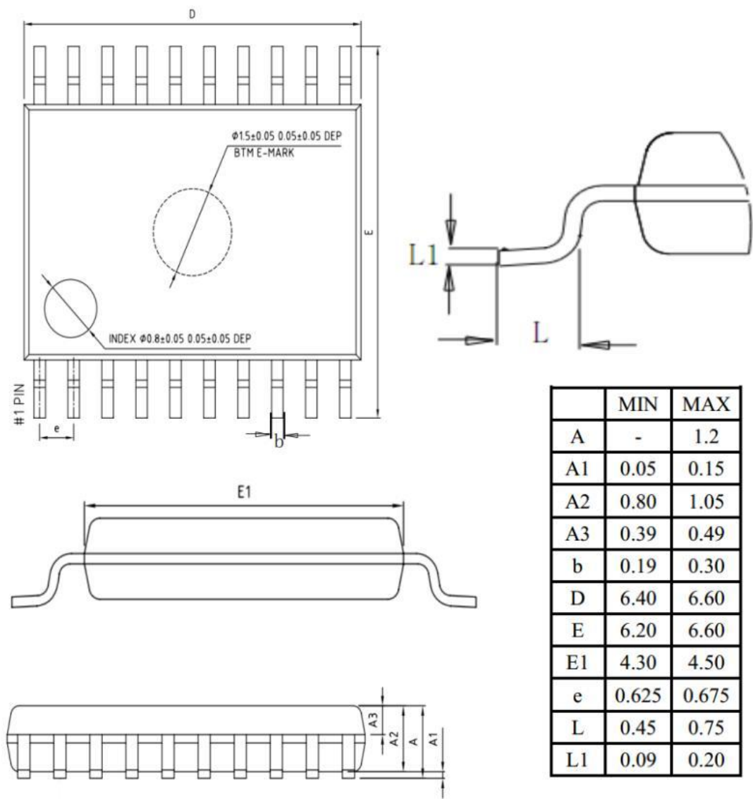
Figure 23- 1 TSSOP20 封装尺寸
