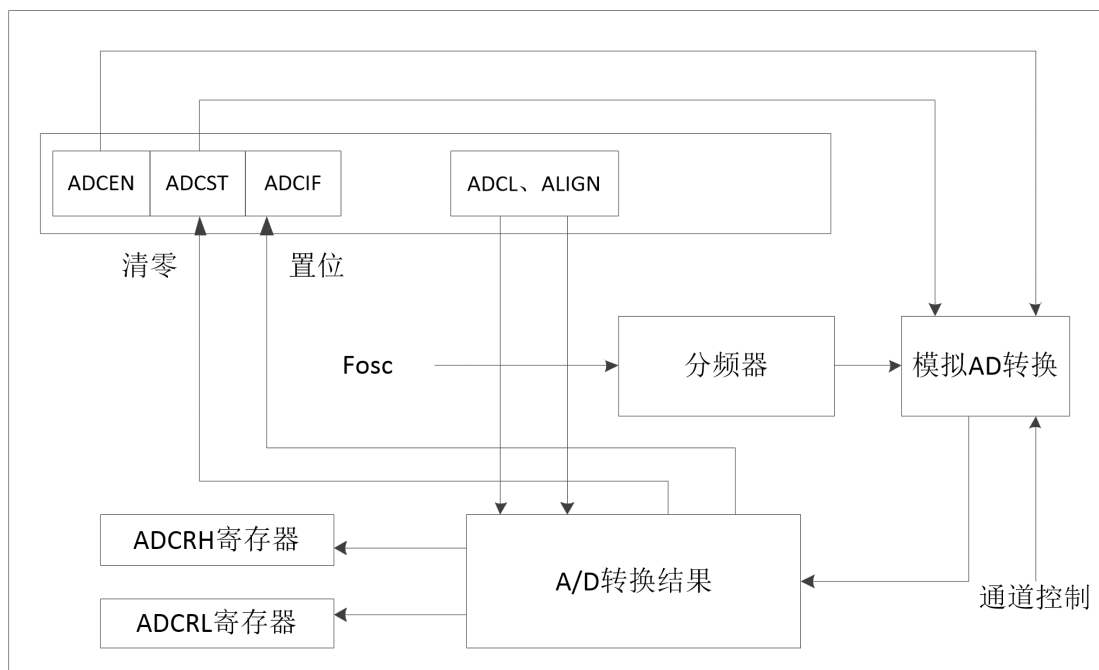
Figure 15-1 ADC 功能框图
