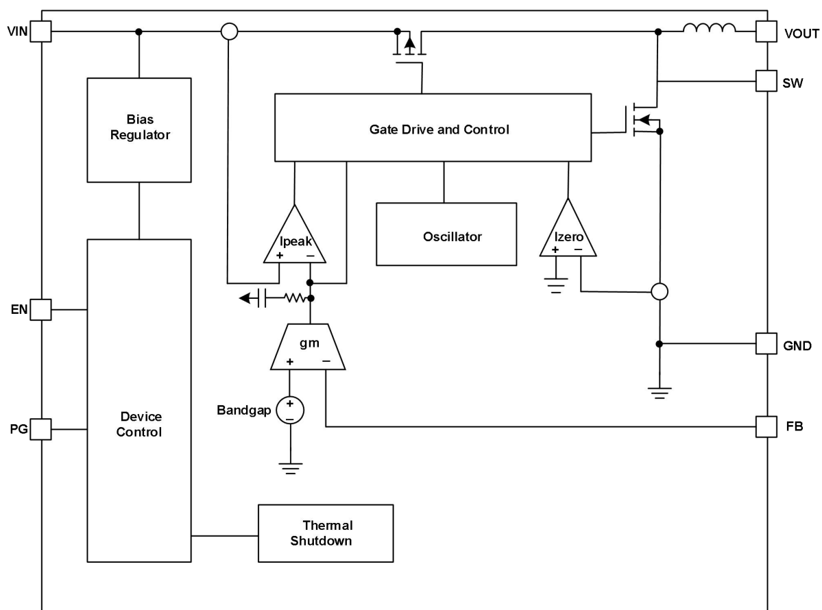
图 2 GM6503A 功能框图
