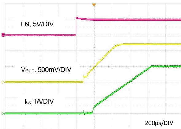
图 13. 启动波形, V_{OUT} = 1.2V , I_O = 3A
