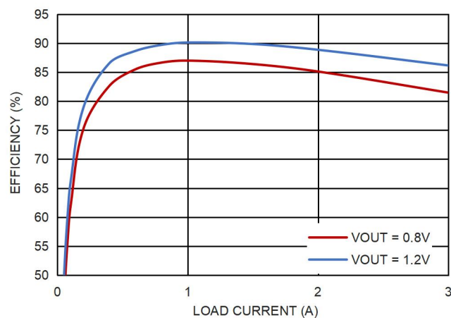
图 4. 效率曲线, V_{IN} = 3.3V
