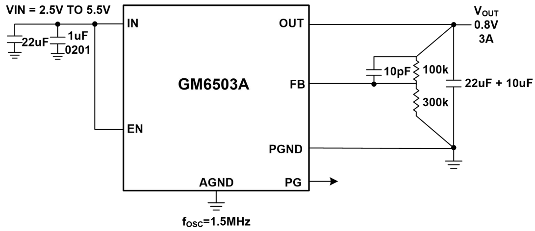
图 17. V_{IN}=3.3V , V_{OUT}=0.8V , I_{LOAD}=3A
