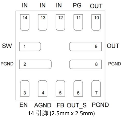
图 3 引脚配置 TOP VIEW
