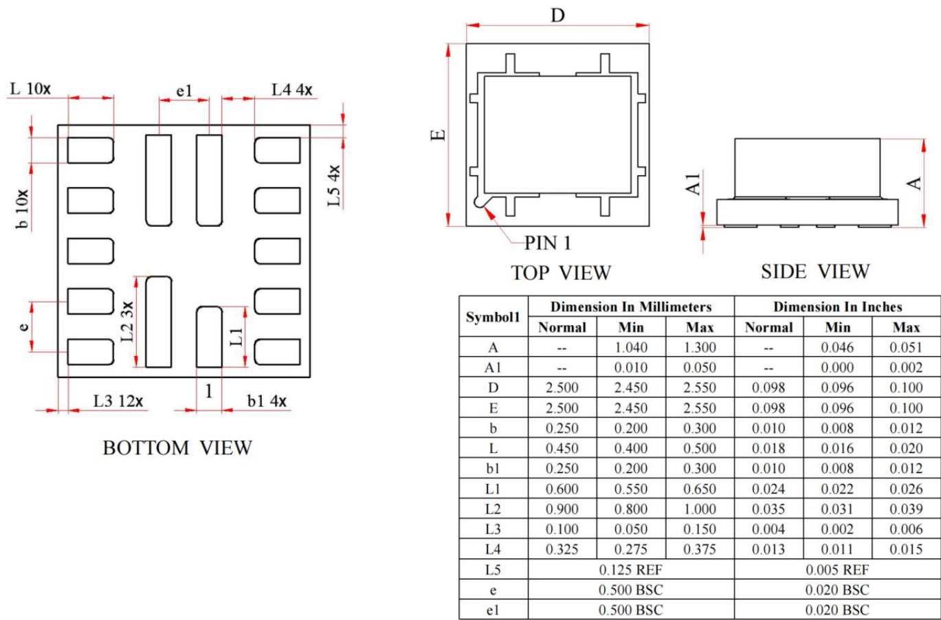
图 18. 14 引脚 LGA (2.5mm x 2.5mm)
