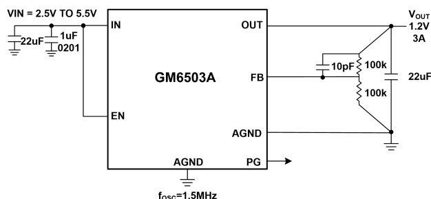
图 1. GM6503A 典型应用
