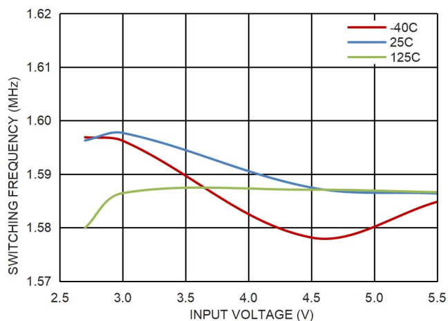
图 7. 频率和输入电压的关系
